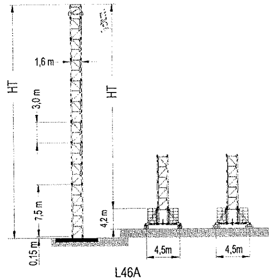
Tower configuration 塔身组成
